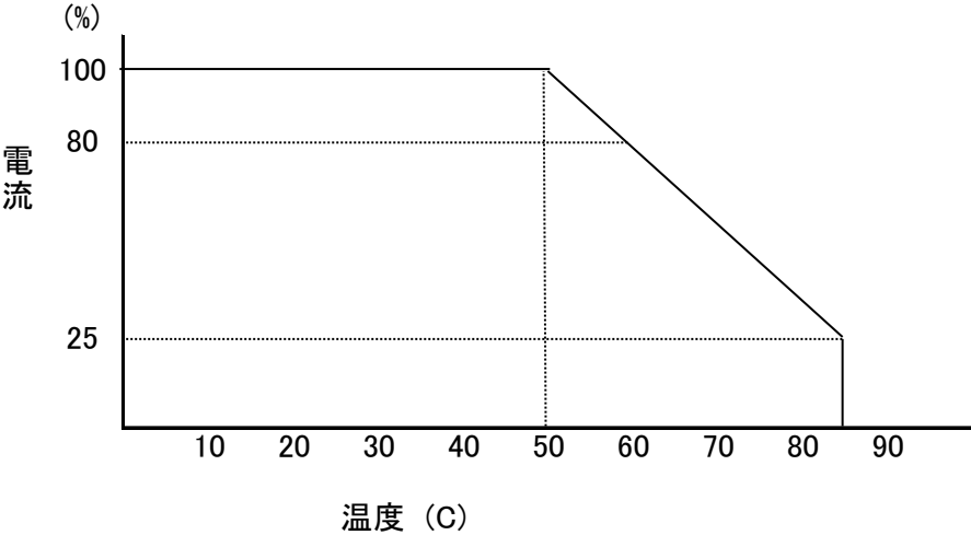
温度ディレーティング表
